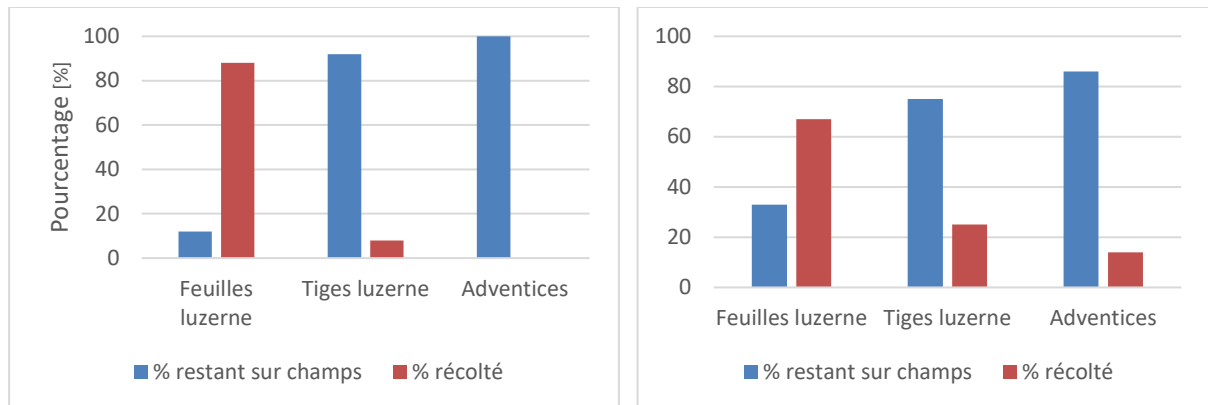
Graphique 1 : Pourcentage d'éléments récoltés et restés au champ avec les deux différents prototypes (à gauche : prototype à dent, à droite : prototype à peigne).
